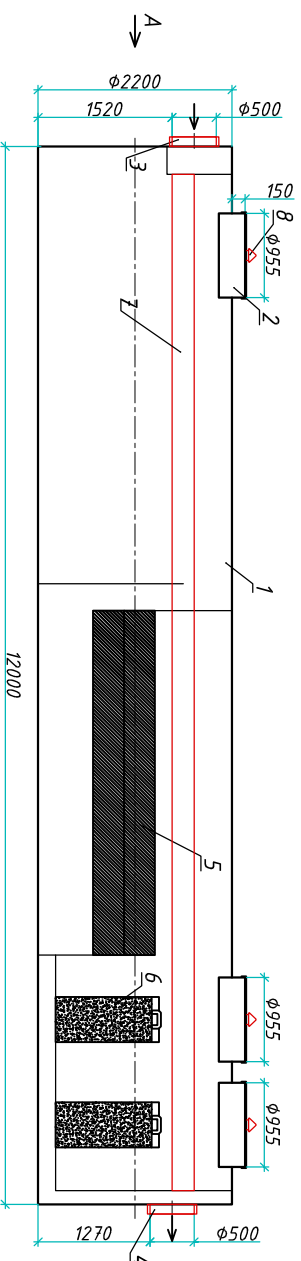
Рәзрәз 1-1
